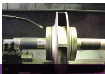
Reparatur einer Welle
